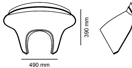
CV11 Variante 2
