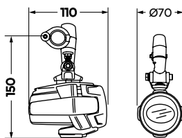
DIMENSIONES
