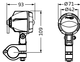
DIMENSIONES
