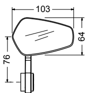
DIMENSIONES
